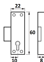
Cerradura vitrina
