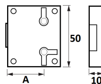
Cerradura armario
